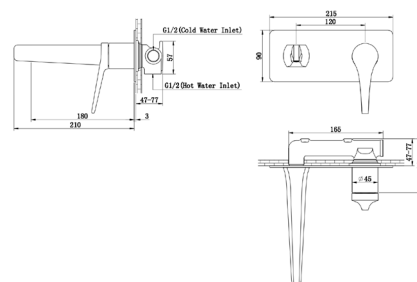
GT Torneira Monocomando para Lavatório Mural CLÁSSICOS
