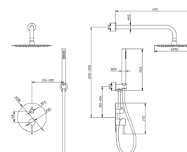
MRT3 Torneira para BanhoDuche (4saidas-2funções) 100% AÇO INOXIDÁVEL AISI 304
